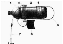
Рис.4. Плавающее жерлицы: 1 - раздаточная камера; 2 - колодезь якоря; 3 - бутылка; 4 - свинец; 5 - грузило; 6 - фанера; 7 - катушка с веревочкой.
